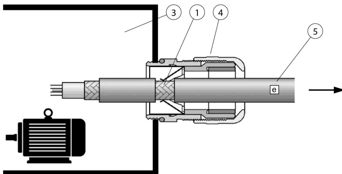
Fig. 37: Conectar pantalla del cable de motor
