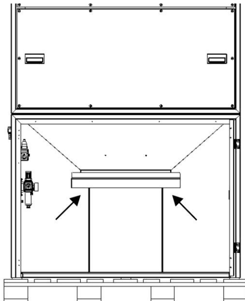
Fig. 19: Elevación del módulo del filtro con una carretilla elevadora
