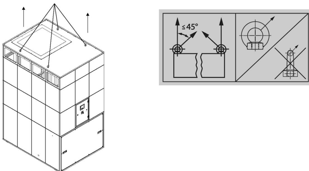
Fig. 10: Elevación del ventilador con grúa
