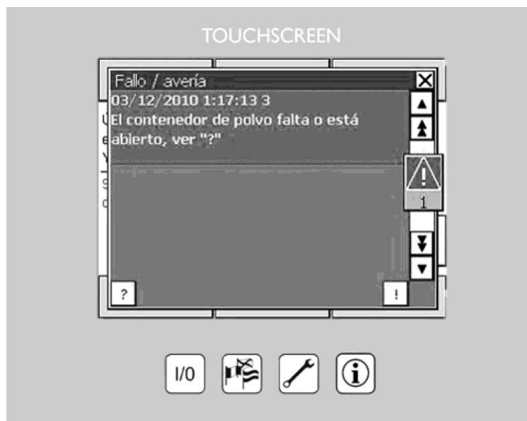
Fig. 56: Mensaje de fallo del depósito colector de polvo
