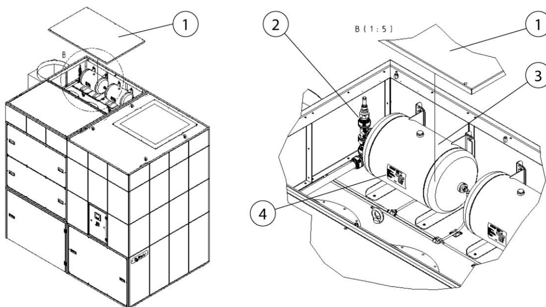
Fig. 74: Acceso depósito de aire comprimido + válvula de seguridad
