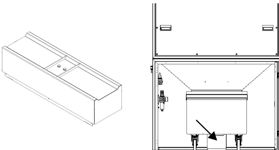
Fig. 24: Fijación del dispositivo de elevación al suelo
