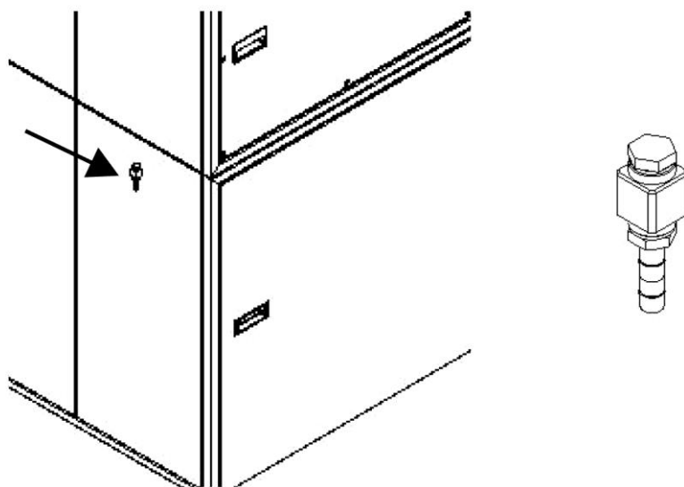
Fig. 28: Conexión de la alimentación de aire comprimido
