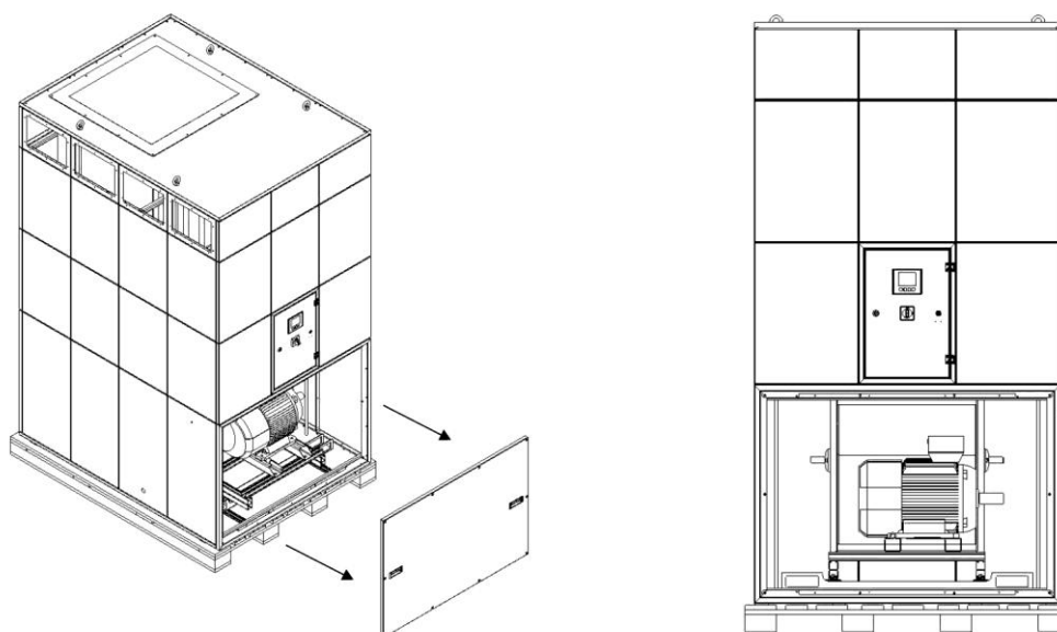
Fig. 9: Abra la puerta de mantenimiento del ventilador
