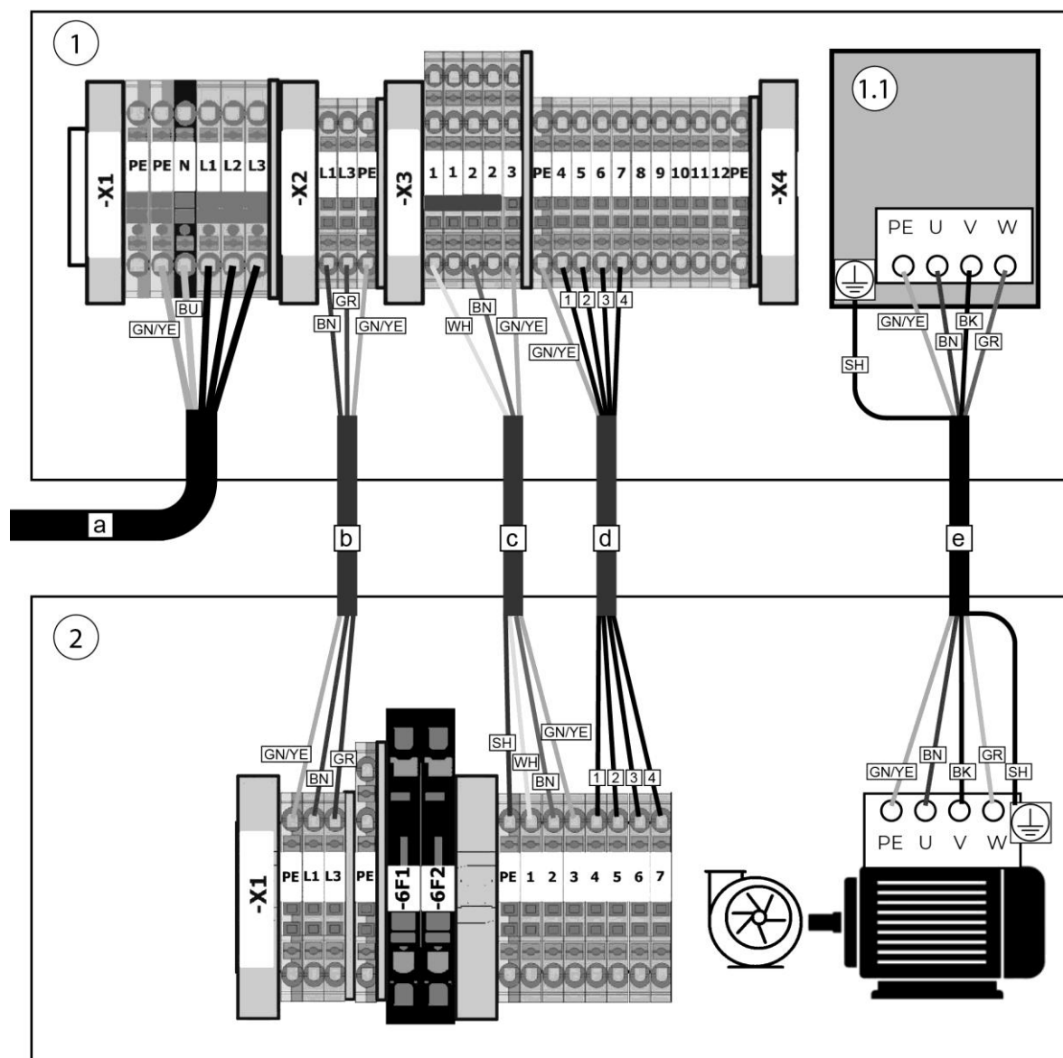
Fig. 35: Esquema de cableado regulación de la potencia de aspiración con producto
