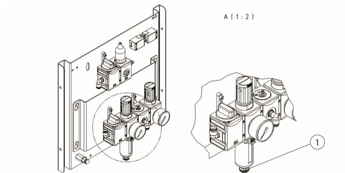
Fig. 71: Válvula de descarga de condensado unidad de mantenimiento de aire comprimido
