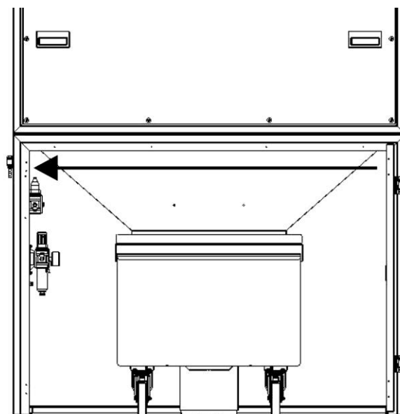
Fig. 25: Tendido del cable a través del canal para cables
