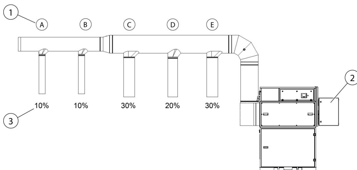
Fig. 54: Ajuste de la regulación de la potencia de aspiración
