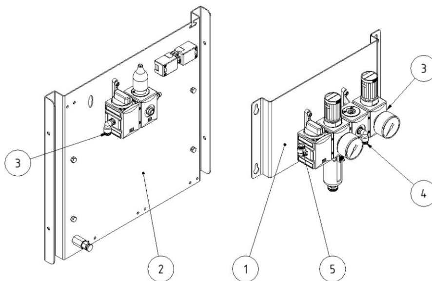
Fig. 31: Unidad de aire comprimido
