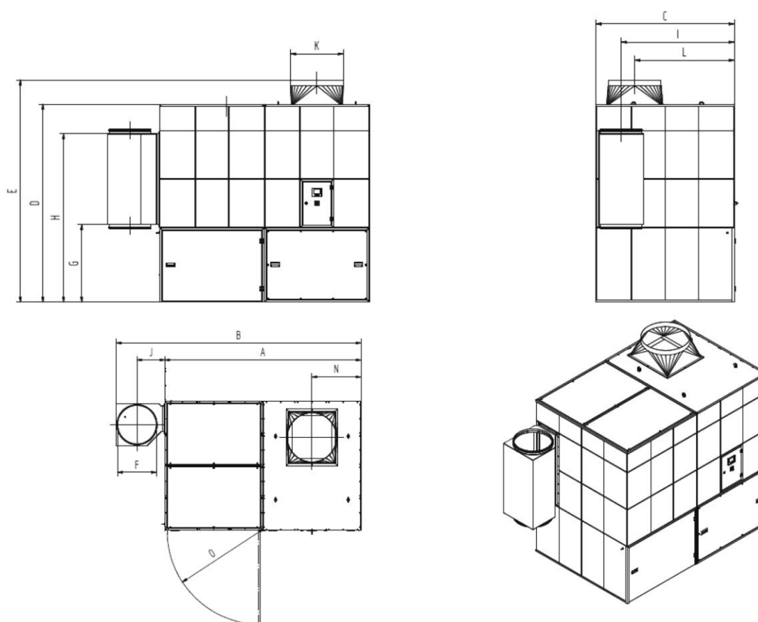
Fig. 75: Hoja de dimensiones 34110
