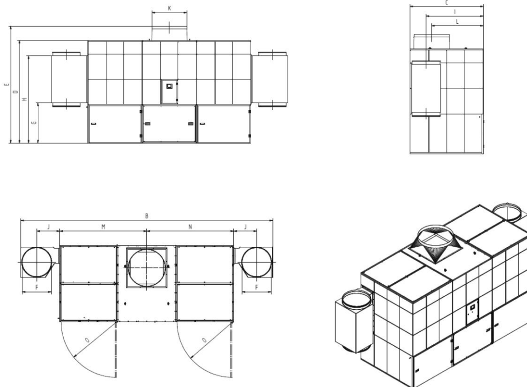
Fig. 78: Hoja de dimensiones 34180
