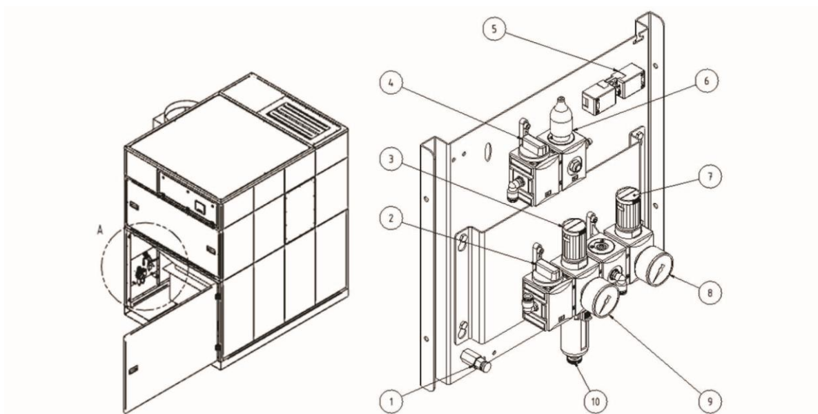
Fig. 27: Unidad de aire comprimido
