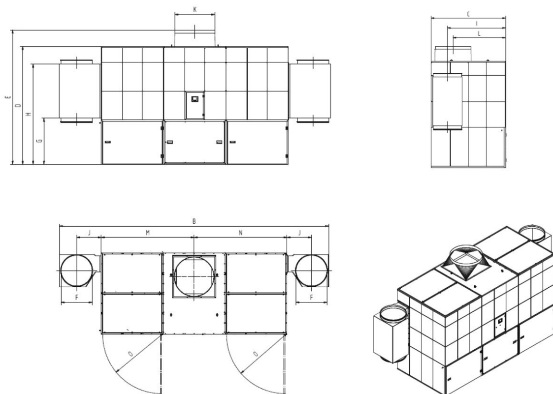
Fig. 79: Hoja de dimensiones 34200 + 34220
