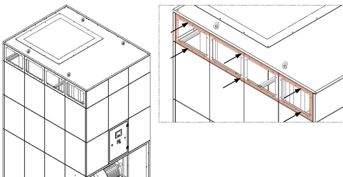
Fig. 12: Paso del aire limpio
