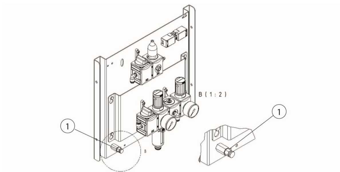
Fig. 70: Válvula de descarga de condensado depósito de aire comprimido
