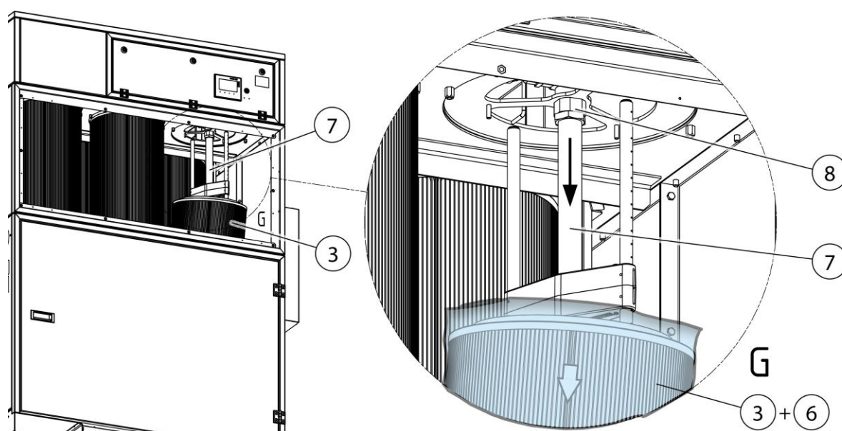
Fig. 63: Desmontar la tobera rotativa
