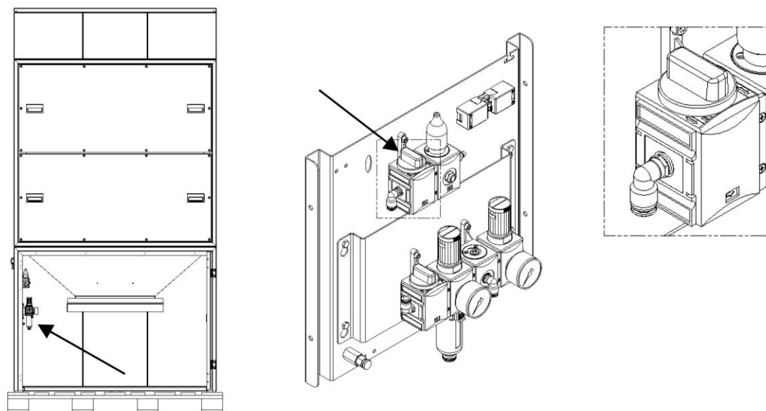
Fig. 14: Válvula de descenso del colector de polvo
