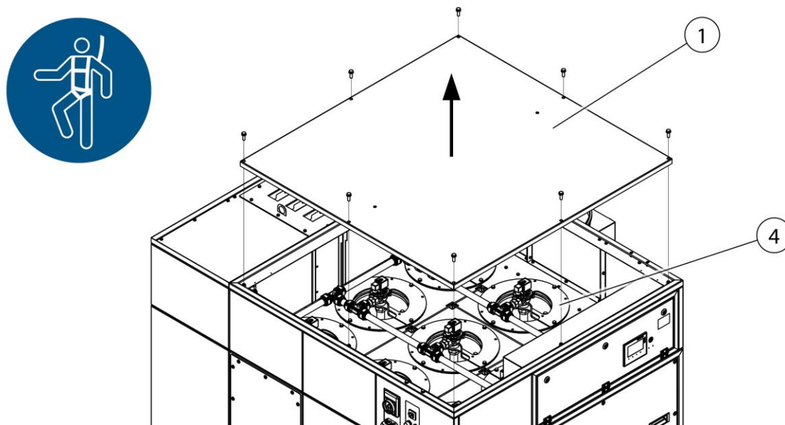
Fig. 64: Sustitución del filtro - desmontar la chapa de tapa
