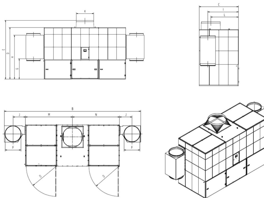
Fig. 77: Hoja de dimensiones 34160
