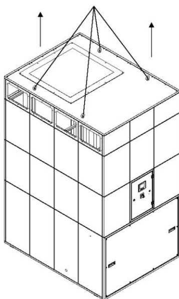
Fig. 18: Elevación del módulo del filtro con grúa
