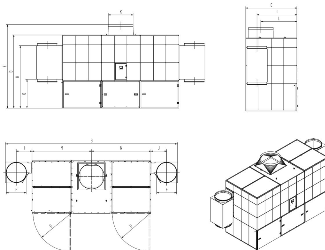
Fig. 80: Hoja de dimensiones 34240 + 34270
