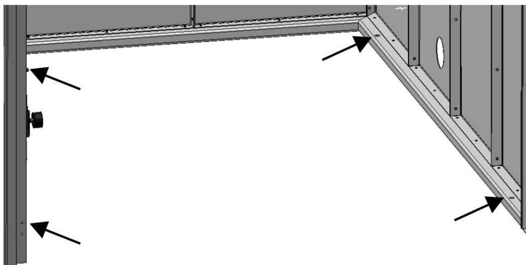
Fig. 23: Fijación del módulo del filtro al suelo
