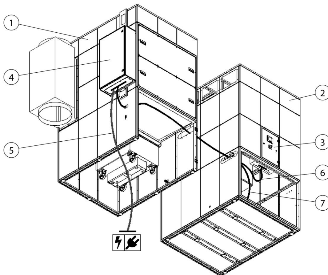
Fig. 33: Ejemplo: Cableado regulación de la potencia de aspiración
