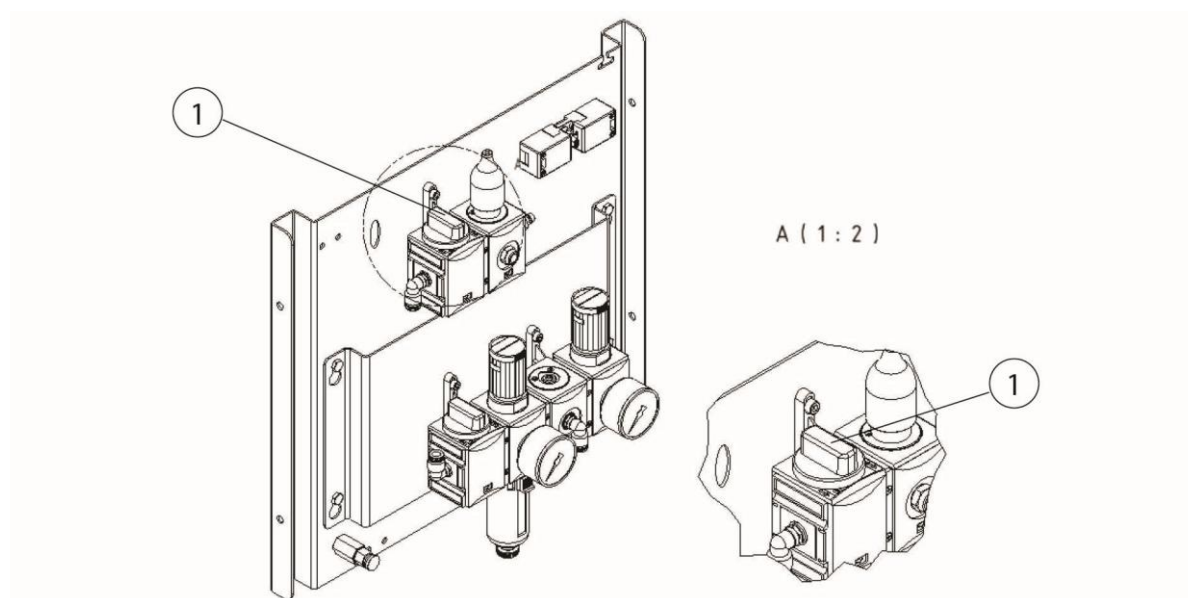
Fig. 55: Válvula de aire comprimido depósito colector de polvo
